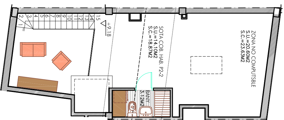
PLANTA SOTACOBERTA
